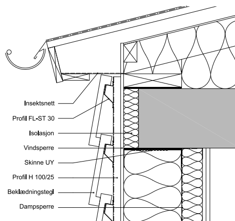
Vertikalsnitt ved gesims
