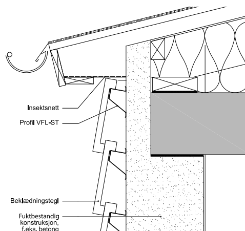
Vertikalsnitt ved gesims
