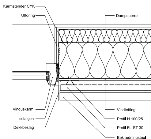
Vertikalsnitt ved vindu
