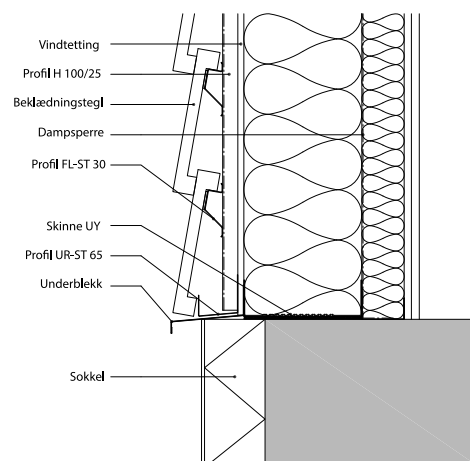
Vertikalsnitt ved sokkel
