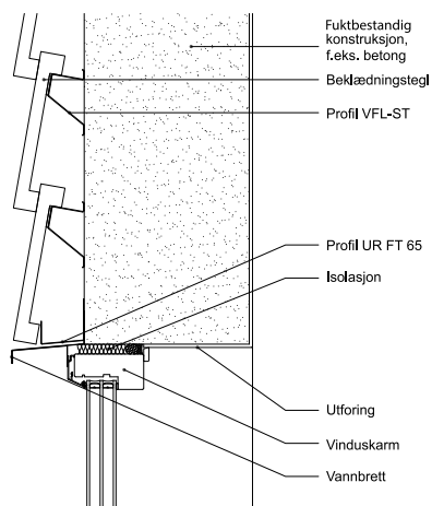
Vertikalsnitt over vindu
