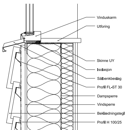
Vertikalsnitt under vindu
