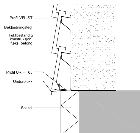
Vertikalsnitt ved sokkel
