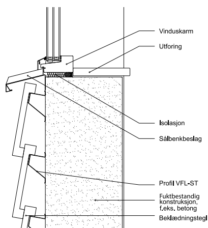
Vertikalsnitt under vindu
